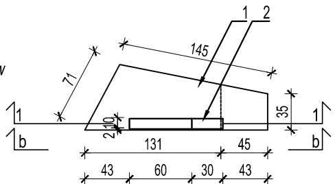
Izgled / View a-a
