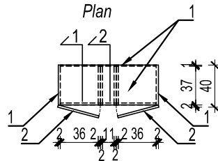
Izgled / View
