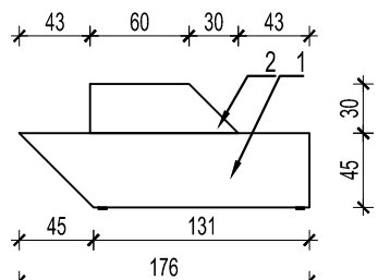
Izgled / View b-b
