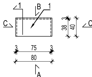
Osnova / Plan
