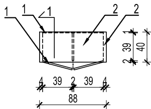
Osnova / Plan
