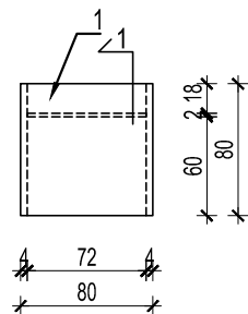
Osnova / Plan
