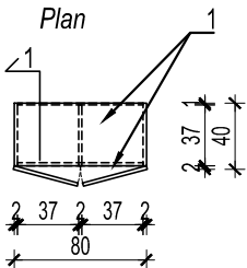
Osnova / Plan
