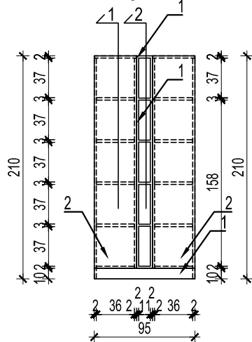
Izgled / View
