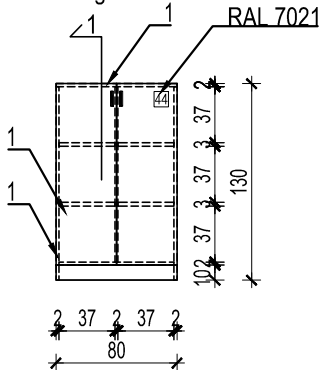
Izgled / View
