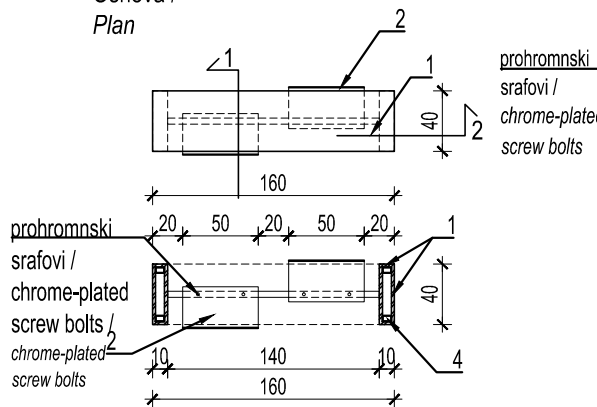
Izgled / View
