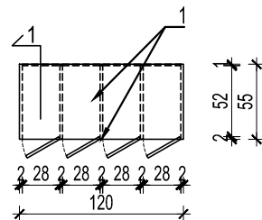
Osnova / Plan
