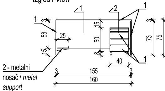
Izgled / View
