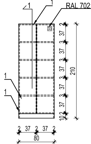
Izgled / View
