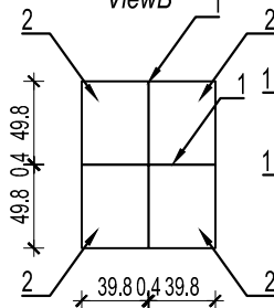
Izgled / ViewB
