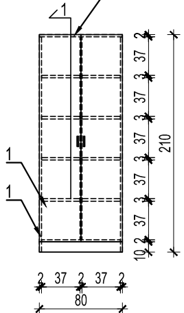
Izgled / View
