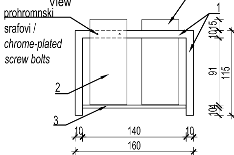
Izgled / View
